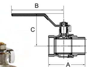
Кран шаровой полнопроходной, ручка-рычаг, Н/В
