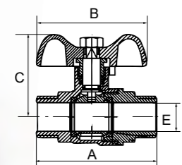
Кран шаровой полнопроходной ручка-бабочка, Н/Н
